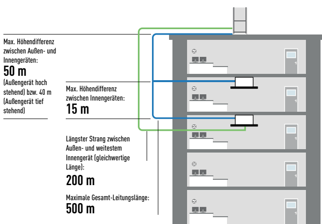
L1 = längster Rohrleitungsstrang, L2 = kürzester Rohrleitungsstrang, L1 - L2 = max. 40 m
