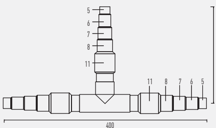
Suction tubing
