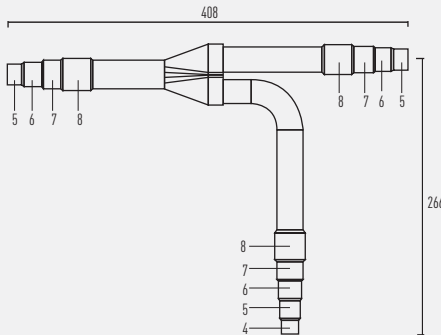
Suction tubing
