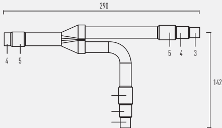
Suction tubing
