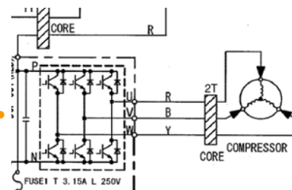
Zaciski sprężarki
