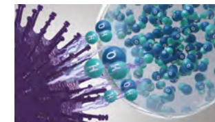
Hydroxylradikale denaturieren die Proteine der Schadstoffe.
