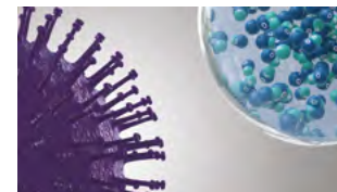
nanoe™ X-Partikel treffen auf Schadstoffe.
