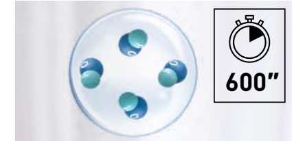
nanoe™ X-Partikel: von Wassertröpfchen umschlossene Hydroxylradikale
