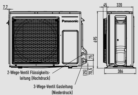
Frontansicht
