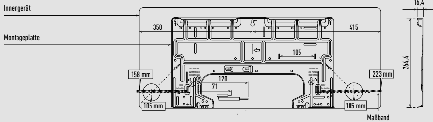
Anordnung von Innengerät und Montageplatte Frontansicht
