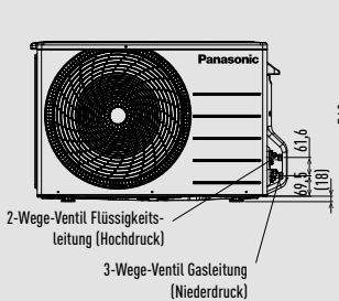
Frontansicht
