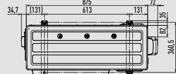
Frontansicht
