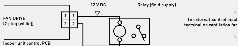
External fan ON / OFF
